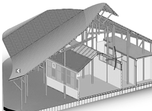
Figura 5: Modelo tridimensional da cobertura. Internet: < www.midiатека.fau.ufrj.br >.
