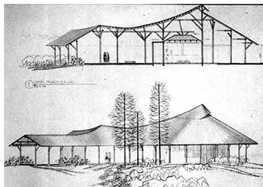
Figura 4: Desenho de cobertura com dispositivo de retirada de ar quente. Foto: Acervo pessoal do arquiteto Severiano Porto.
